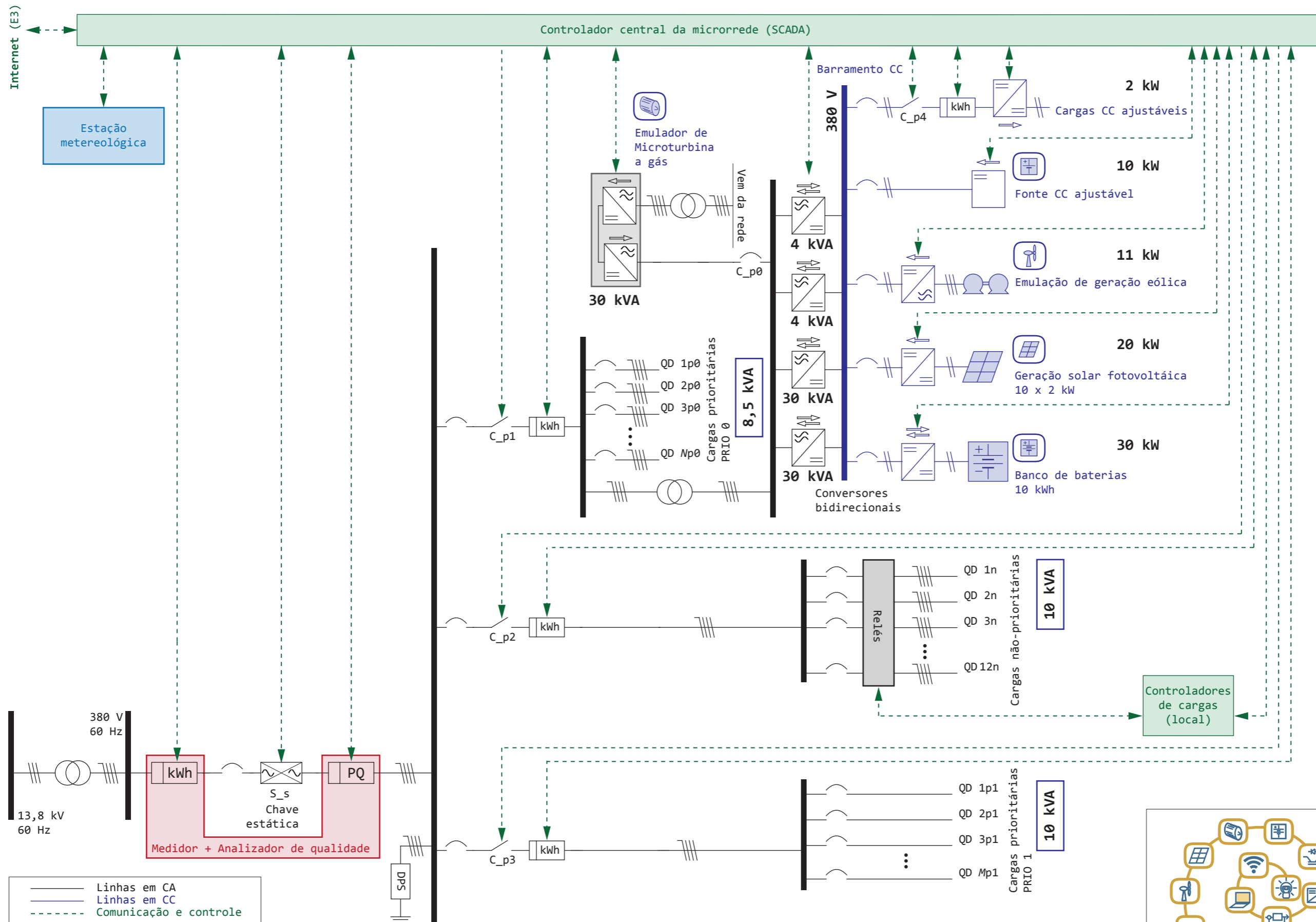
Projeto elétrico: Diagrama básico
